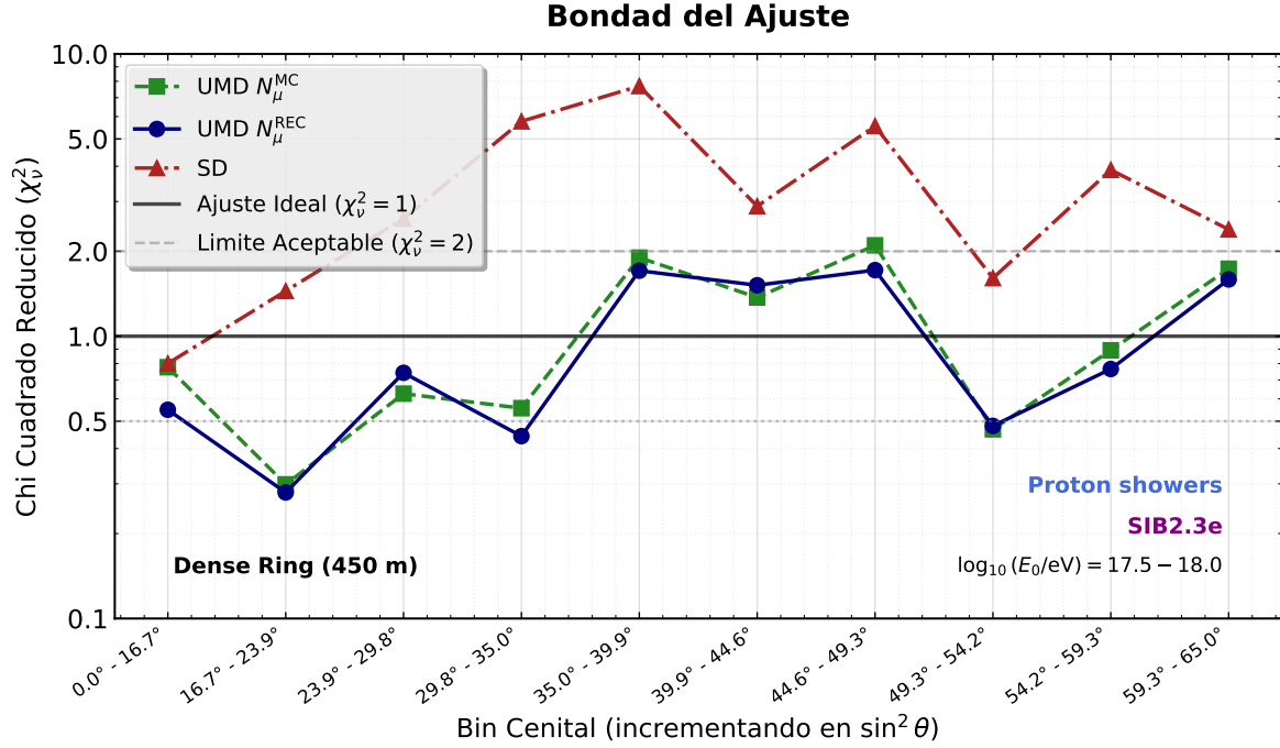
Figura 5.3: Bondad de ajuste \chi^2 para los bins cenitales. Se observa que los ajustes del UMD (REC y MC) se mantienen cercanos a la unidad, mientras que el SD presenta valores elevados debido a la alta precisión estadística de la muestra.
